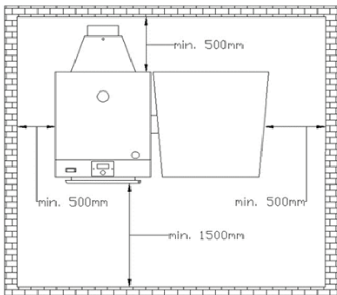
Рис.3 Установка котла в котельной
