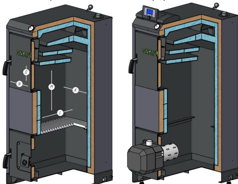
Рис.1 Разрез котла SAKOVICH PELLET STANDART
