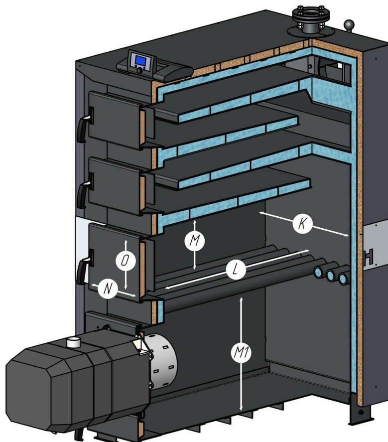
Рис.1 Разрез котла SAKOVICH PELLET MAX 150кВт.
