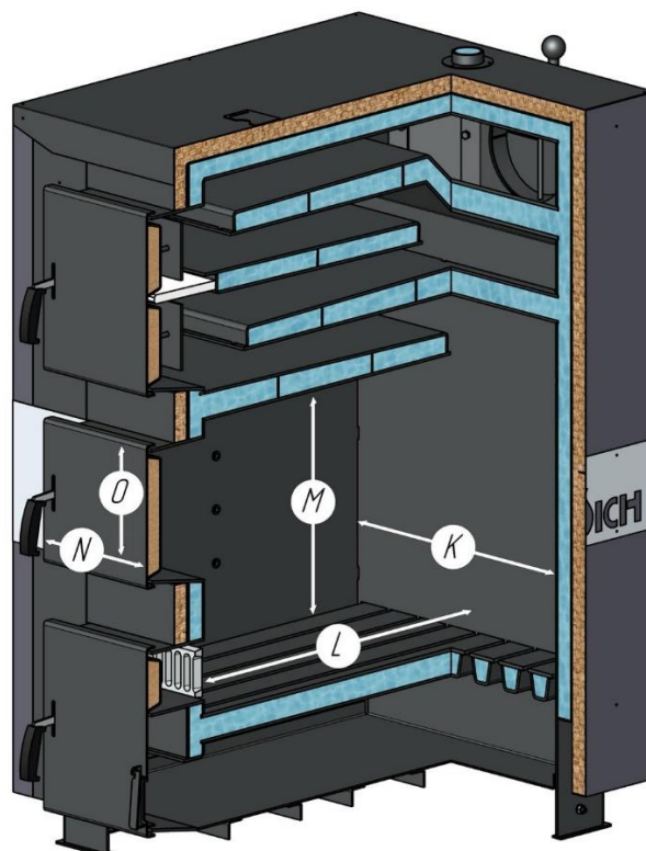
Рис.1 Разрез котла SAKOVICH MAX 99кВт
