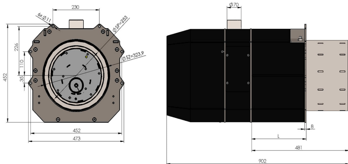
Рисунок № 16 Размеры горелки 200kW.
