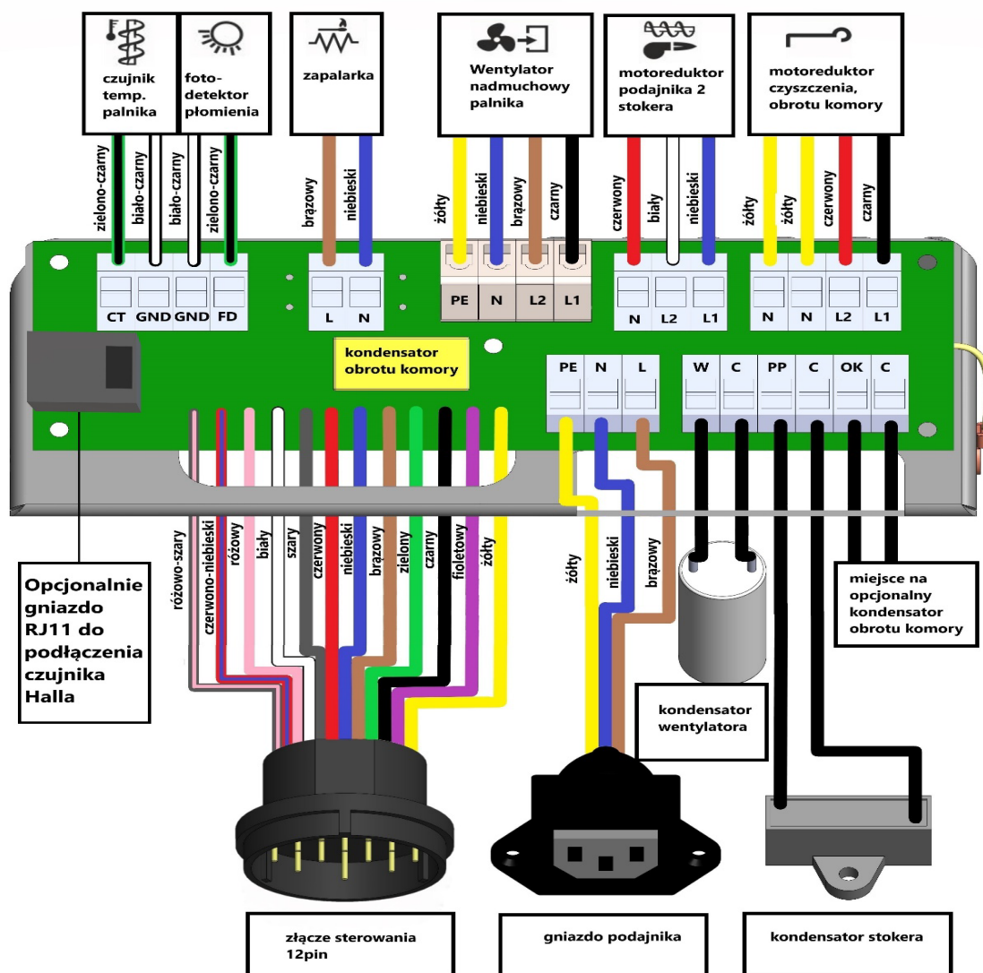
Рисунок № 14 Электрическая схема горелки.
