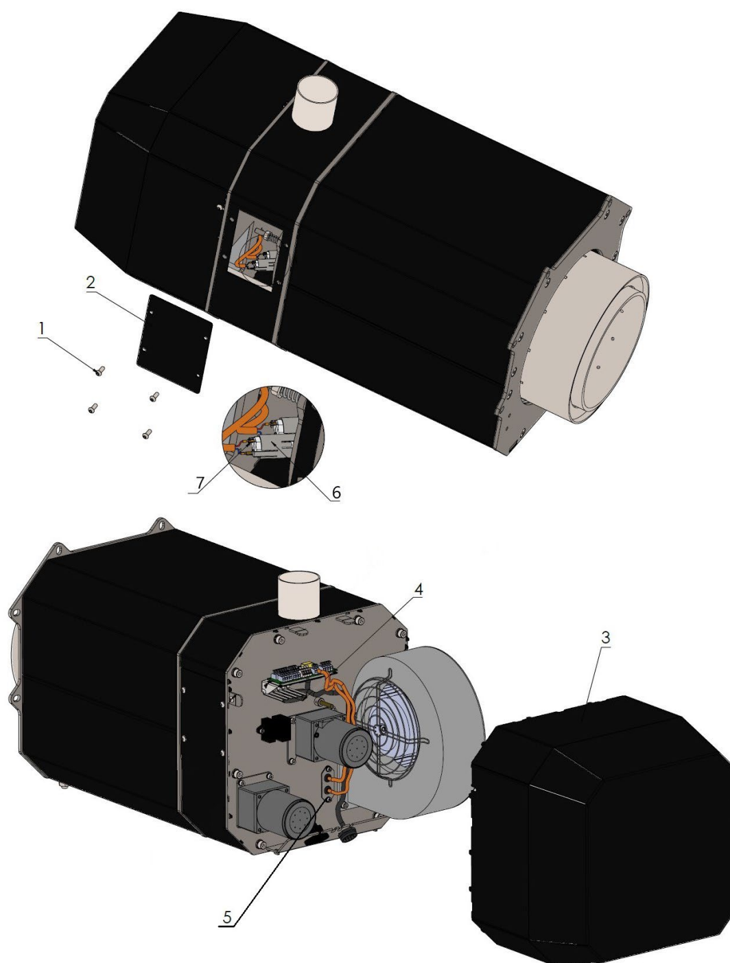
Рисунок № 8 Замена воспламенителя.
