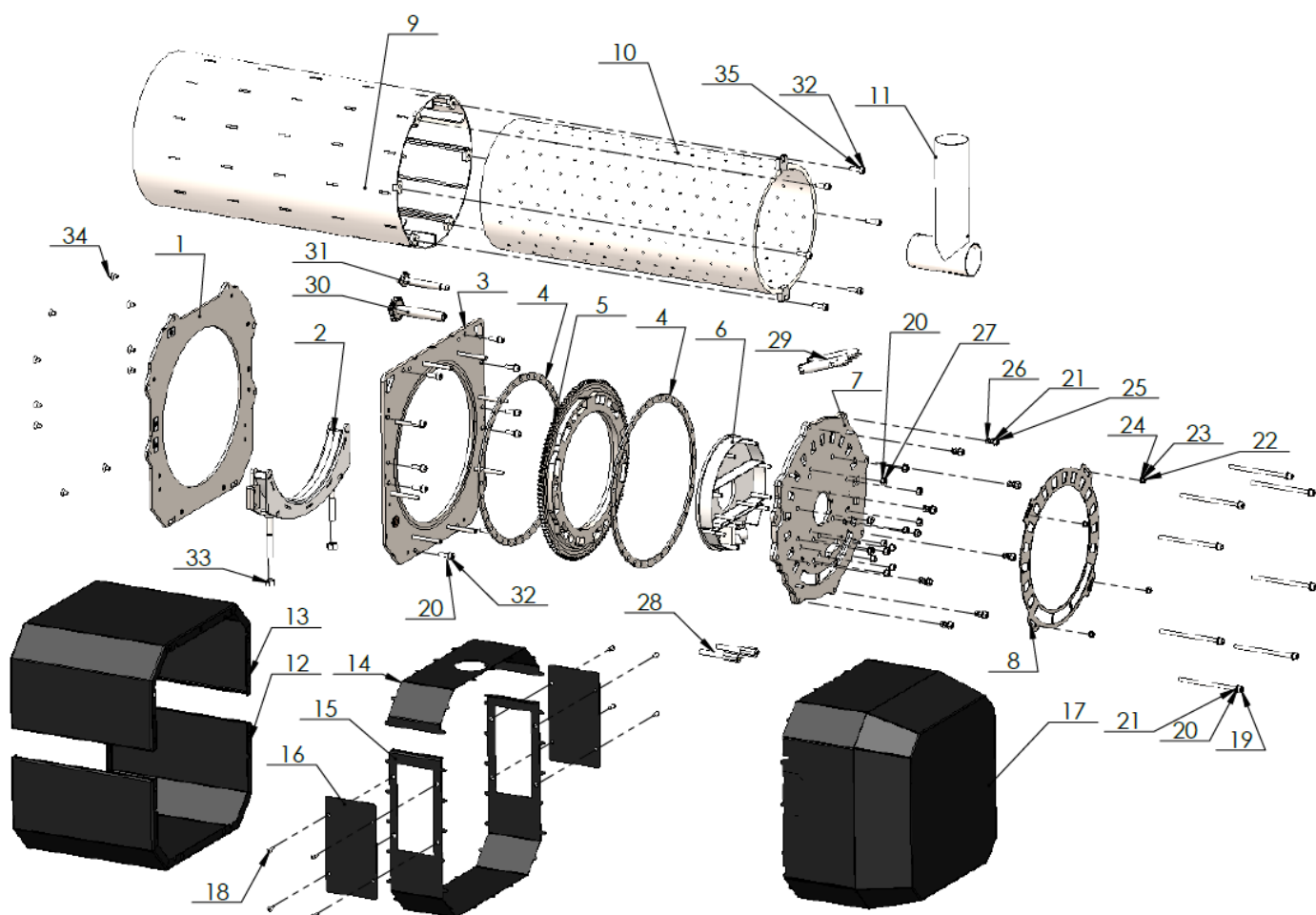
Рисунок № 7. Компоненты корпуса горелок 150kW,200kW,250kW.
