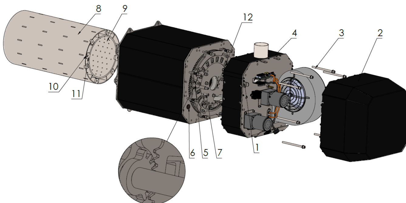
Рисунок № 10 Очистка камеры вентилятора.
