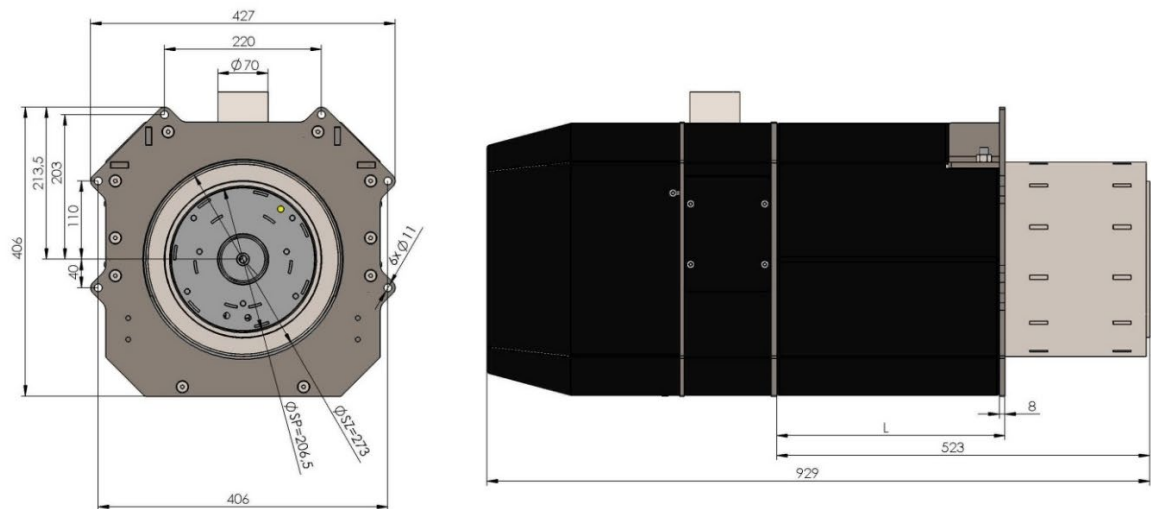
Рисунок № 15 Размеры горелки 150kW.
