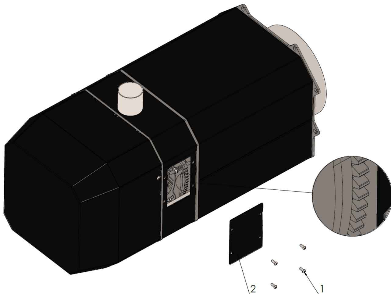
Рисунок № 11 Смазка подшипников камеры сгорания.
