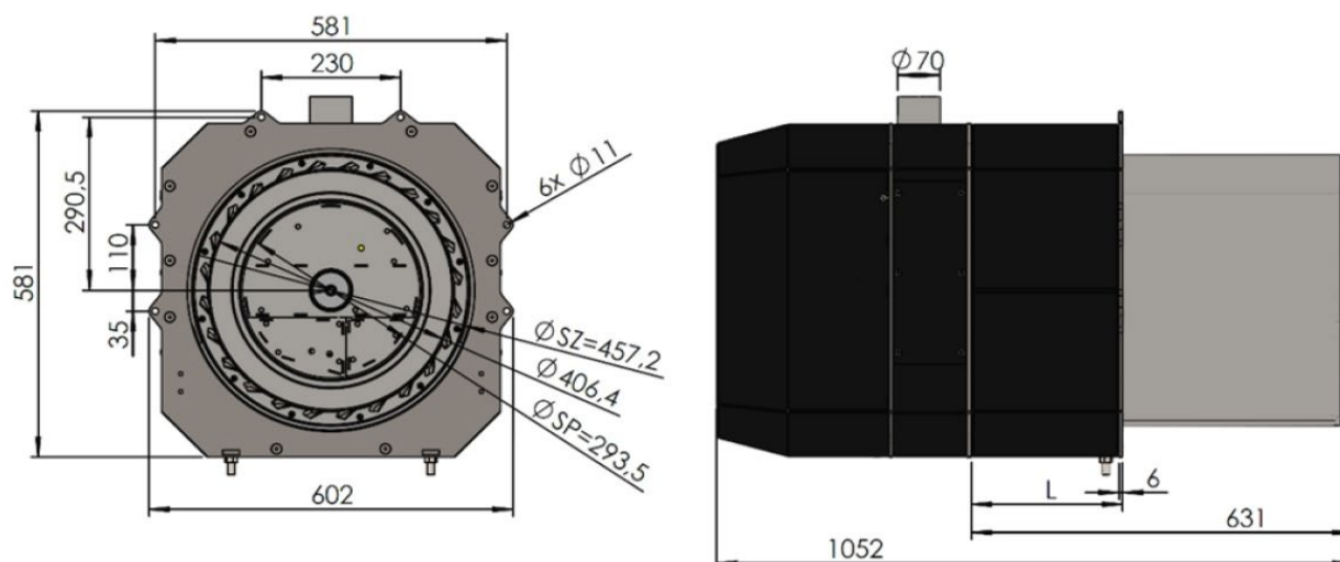
Рисунок № 18. Размеры горелки 300 kW.
