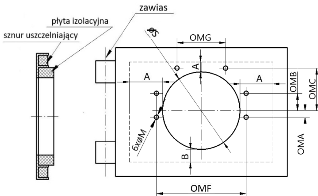
Рисунок № 5. Вырез в двери для установки горелки.
