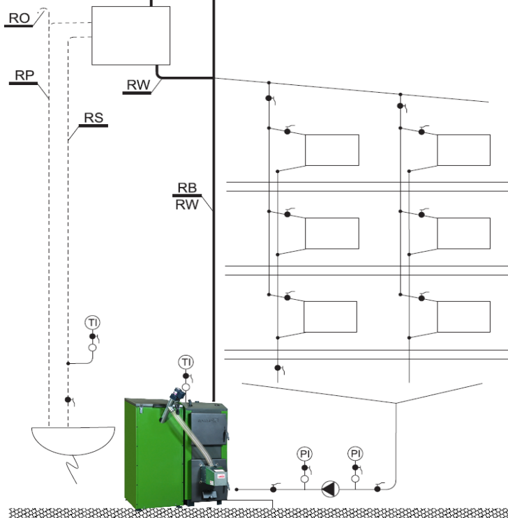
Рис. 5. Примерная схема обеспечения установки водяного отопления оснащенного одним котлом, насос установлен на возврате (согласно PN-91/B-02413).
