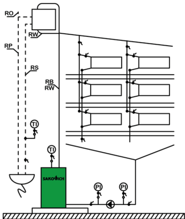
Рис. 56. Пример схемы открытой системы водяного отопления, насос установлен на возврате
