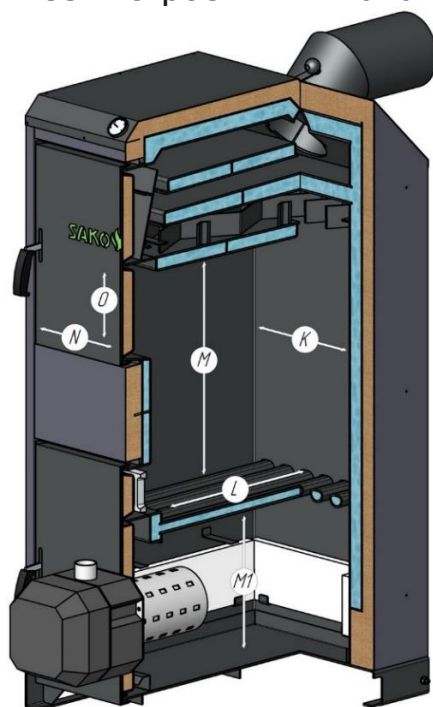
Рис.1 Разрез котла SAKOVICH PELLET UNIVERSAL 50kW
