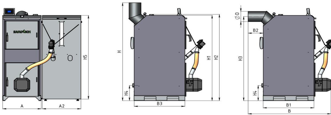
Рис.2 Размеры котла SAKOVICH PELLET UNIVERSAL
