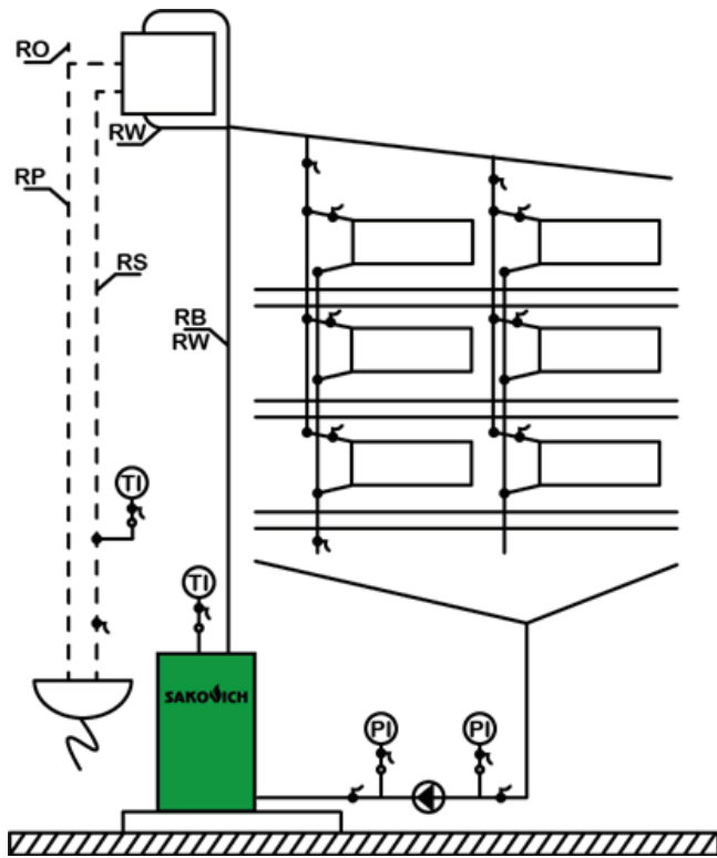
Рис. 5. Пример схемы открытой системы водяного отопления, насос установлен на возврате
