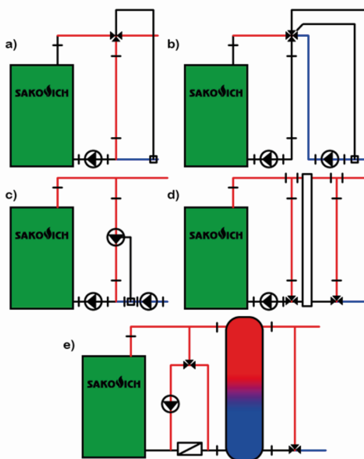
Рис 4. Рекомендуемые схемы соединения котла с системой отопления:
