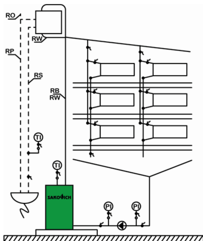
Рис. 5. Пример схемы открытой системы водяного отопления, насос установлен на возврате
