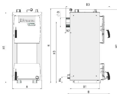
Рис.2 Размеры котла PRAMEN GREEN
