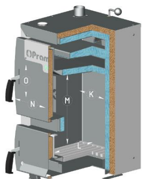
Рис.1 Разрез котла PRAMEN GREEN
