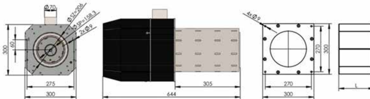
Рис. 25. Вид горелки 15-70 кВт
