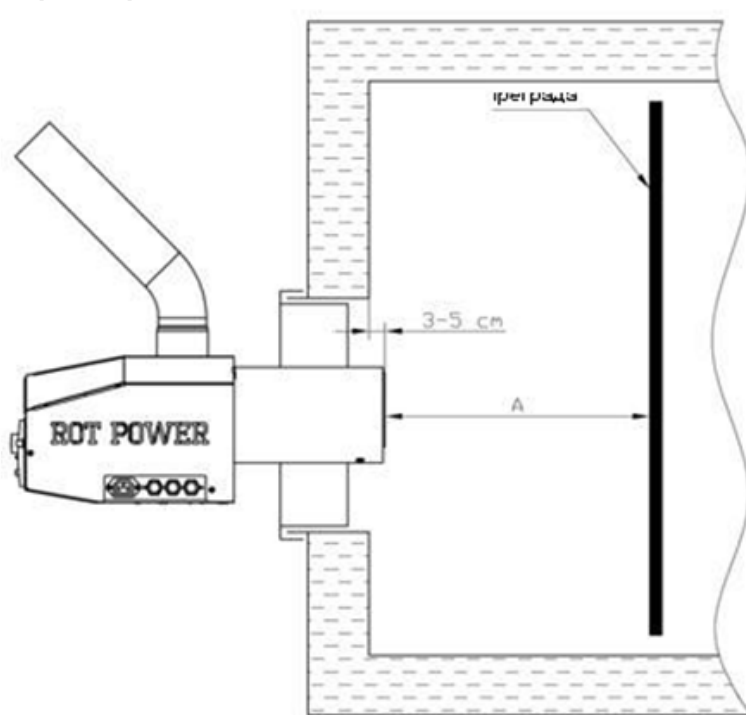
Рис. 8. В камере сгорания котла в боковом поперечном сечении.
