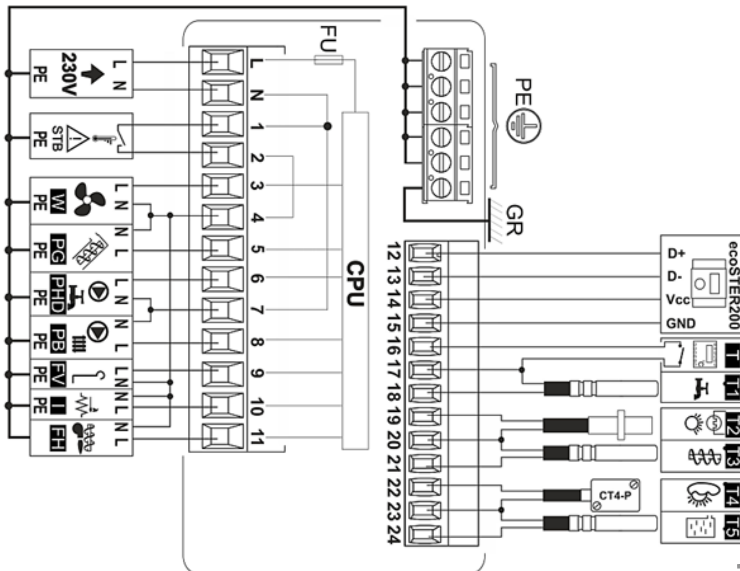
Электрическая схема регулятора есоМАХ 350Р
