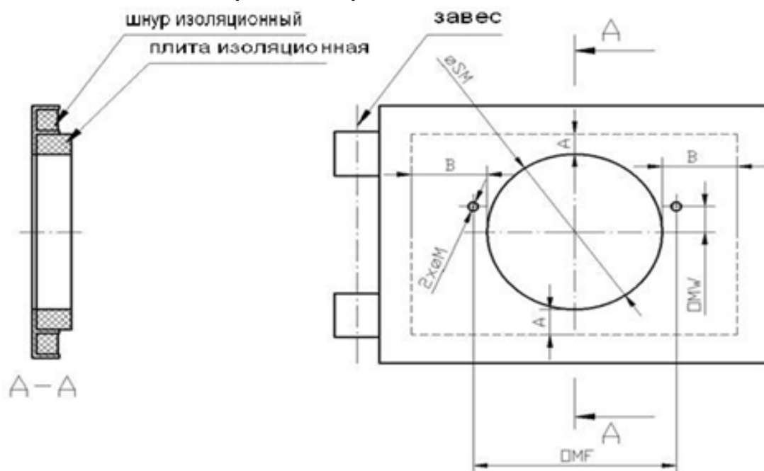
Рис. 4. Схема монтажных отверстий для горелки с монтажной пластиной для горелок: 3-10 кВт, 4-16 кВт, 5-20 кВт, 6-26 кВт, 8-36 кВт.
