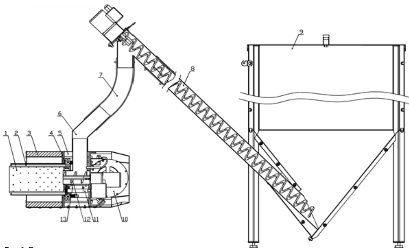
Рис.1. Принципиальная схема горелки
