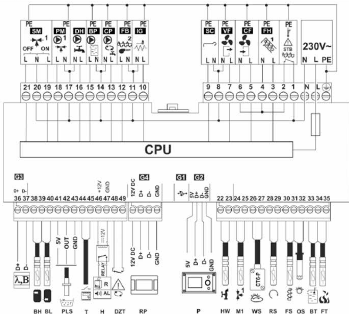
Электрическая схема регуляторов еsoMAX 860P и еsoTOUCH 860P.
