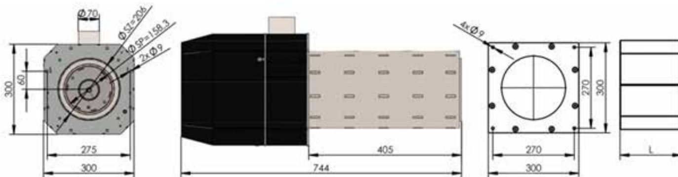
Рис. 26. Вид горелки 20-100 кВт
