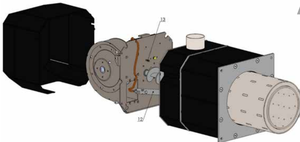
Рис. 12. Очистка трубы воздуходувки горелки 15-70 кВт, 20-100 кВт - вид 2.
