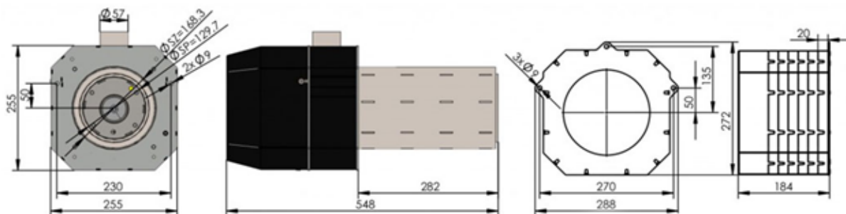
Рис. 24. Вид горелки 10-50 кВт
