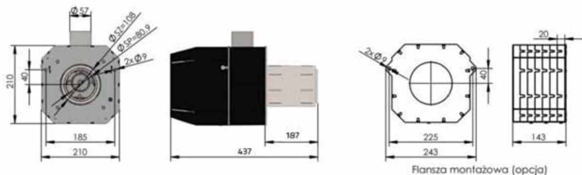
Рис. 19. вид горелки 3-10 кВт
