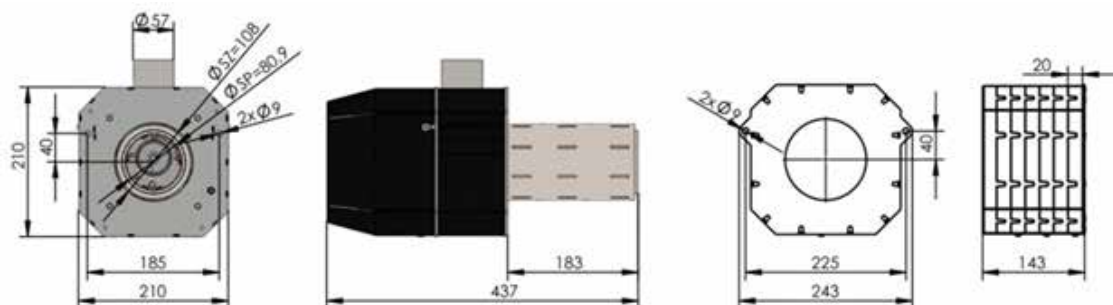
Рис. 20. вид горелки 4-16 кВт
