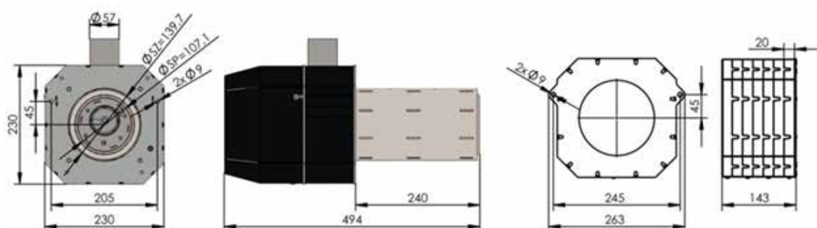
Рис. 23. Вид горелки 8-36 кВт
