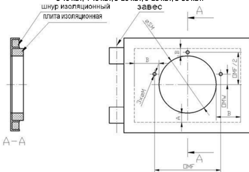
Рис. 5. Схема монтажных отверстий для горелки с монтажной пластиной для горелки 10-50 кВт.
