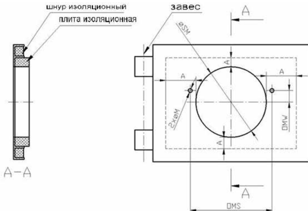
Рис. 3. Схема монтажных отверстий для горелок: 4-16 кВт, 5-20 кВт, 6-26 кВт, 8-36 кВт, 10-50 кВт.
