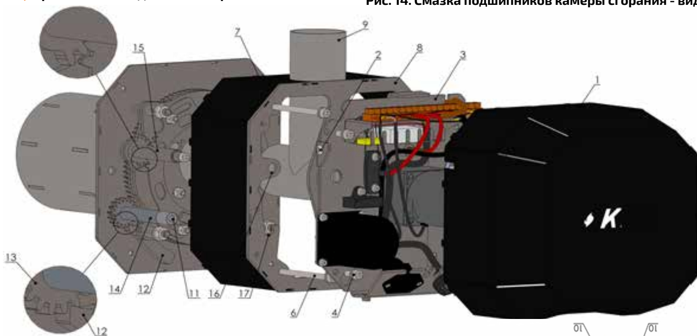
Рис. 14. Смазка подшипников камеры сгорания - вид 1.
