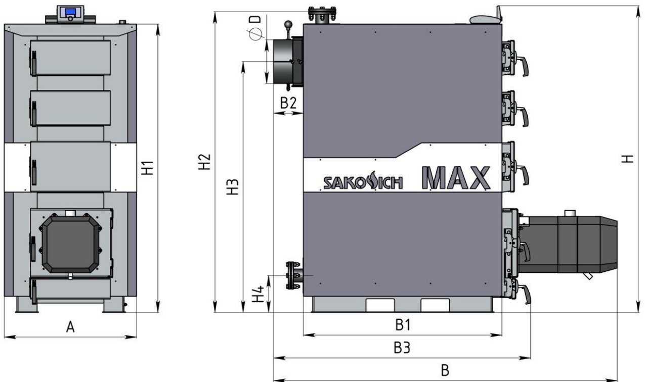
Рис.2 Размеры котла SAKOVICH PELLET MAX 150кВт.
